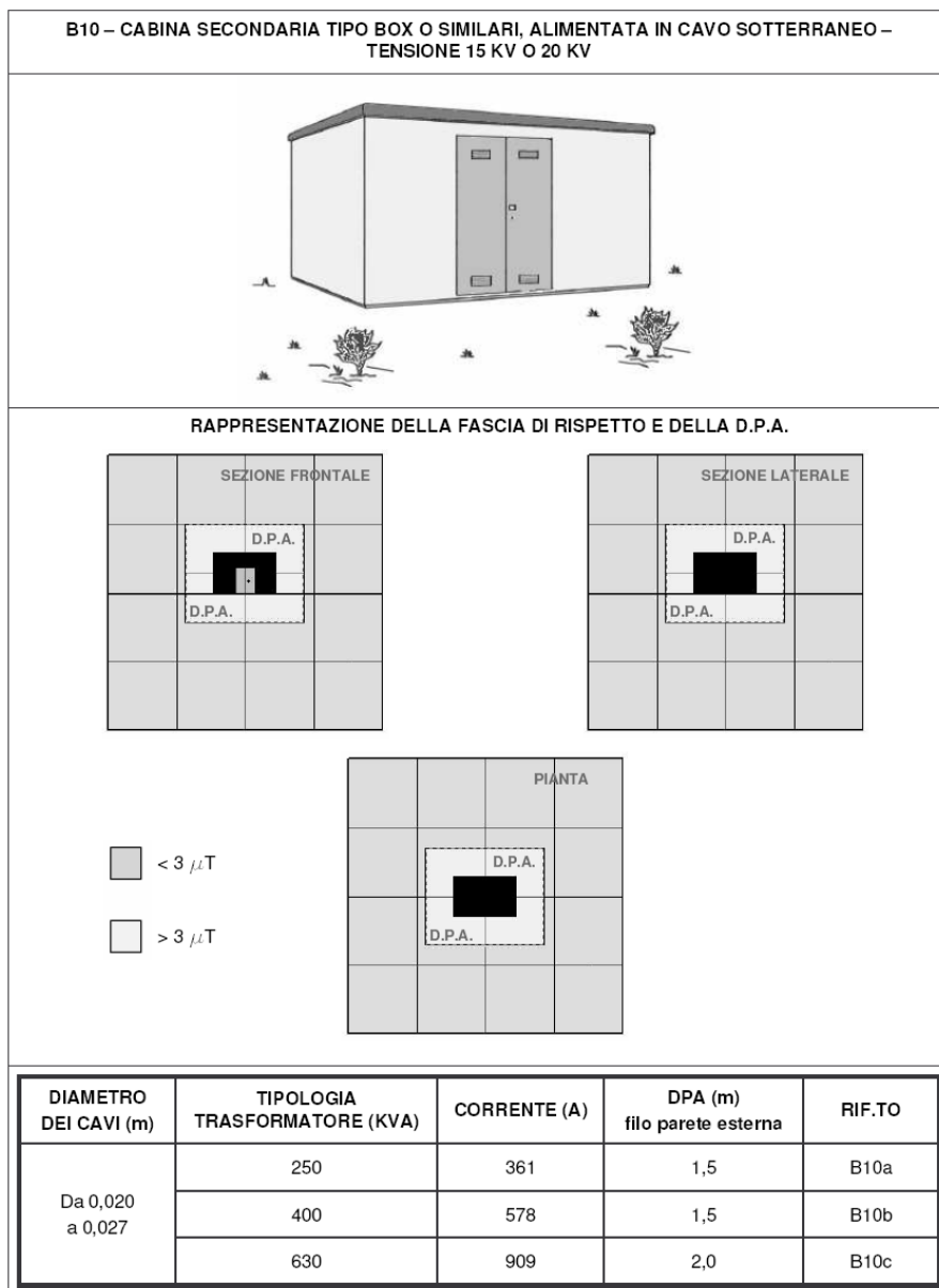
Figura 2 - cabina secondaria
