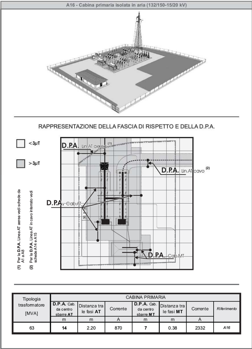
Figura 1 – Cabina primaria (tipologie standard individuate da ENEL)
