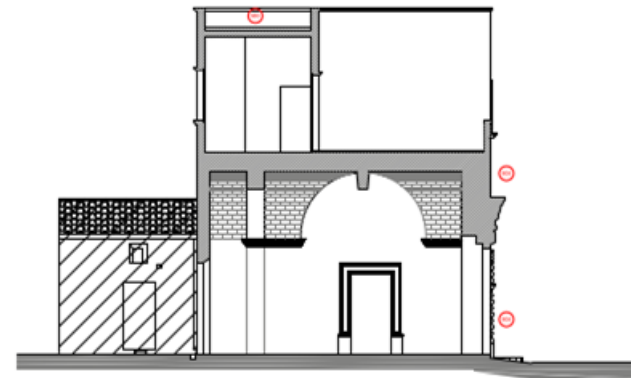
SEZIONE B-B
