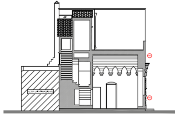
SEZIONE D-D
