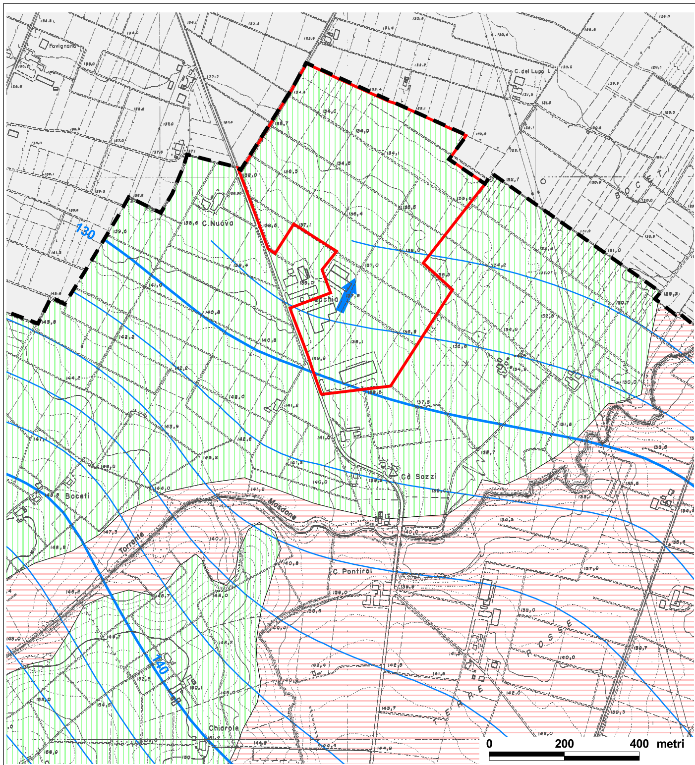
TAV. 4b - CARTA IDROGEOLOGICA
