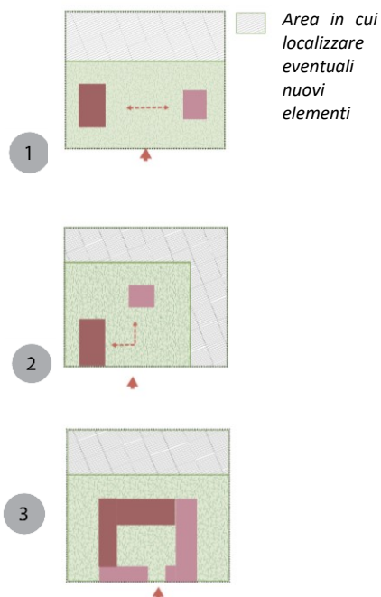
Fig. 1.2.1 Schemi di corte - 1. Aperta ad elementi giustapposti con abitazione e stalla-fienile che si fronteggiano (schema tipico della pianura modenese); 2. Aperta ad "L" con accesso frontale. 3. Chiusa
