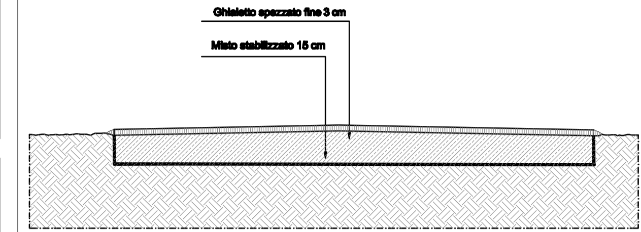
SCALA 1:20
