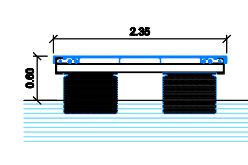
SEZIONE TRASVERSALE (scala 1:50)
