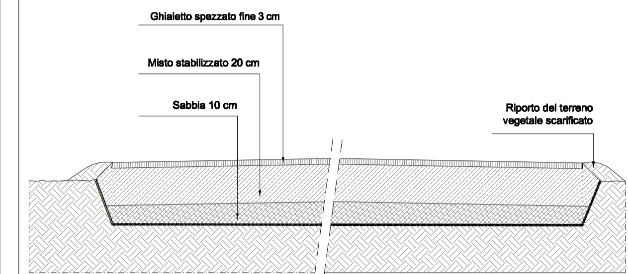
SCALA 1:20
