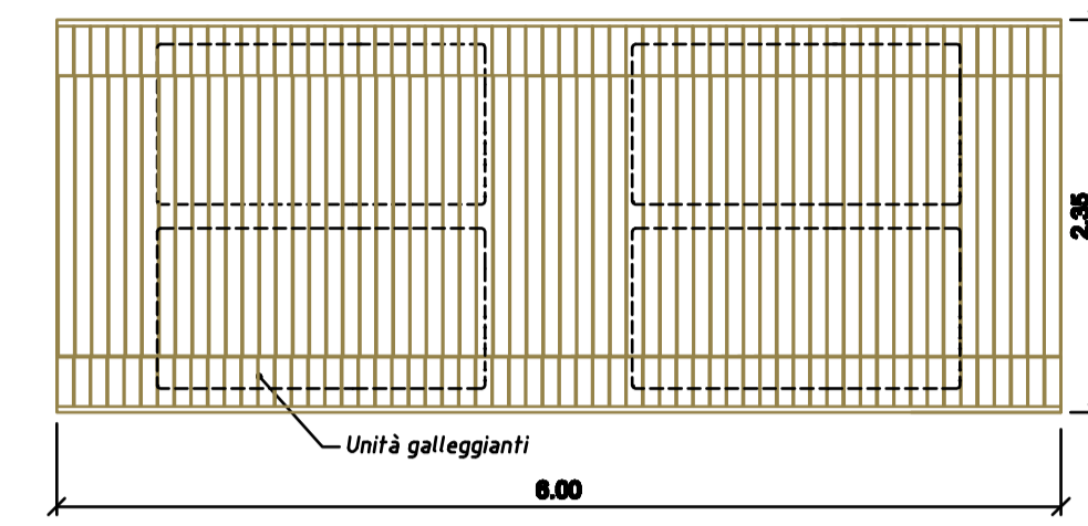
PIANTA (scala 1:50)
