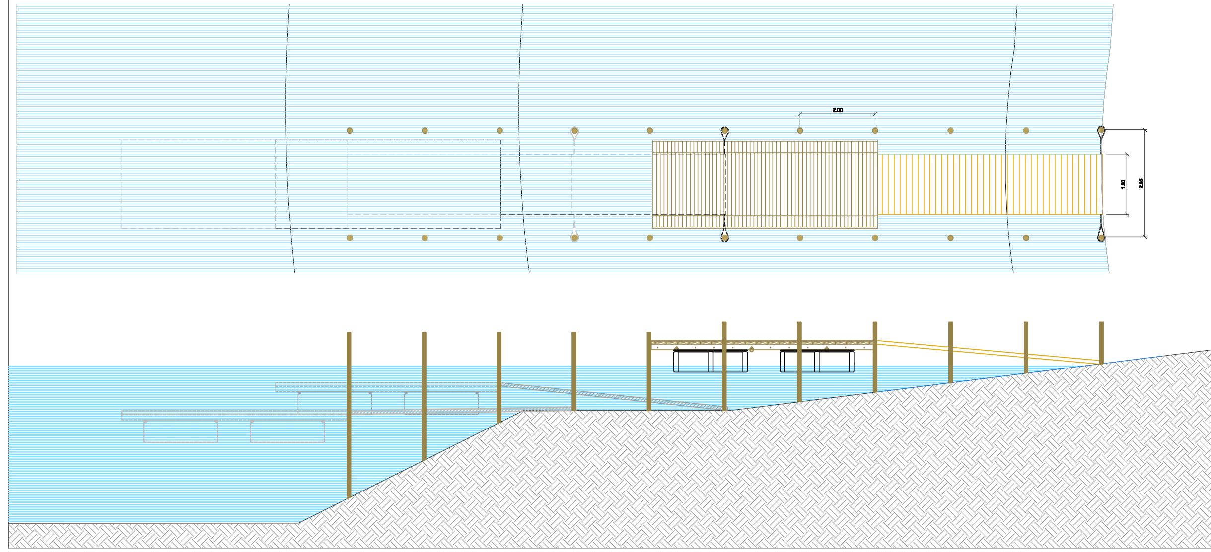
PONTILE GALLEGGIANTE (scala 1:100)
