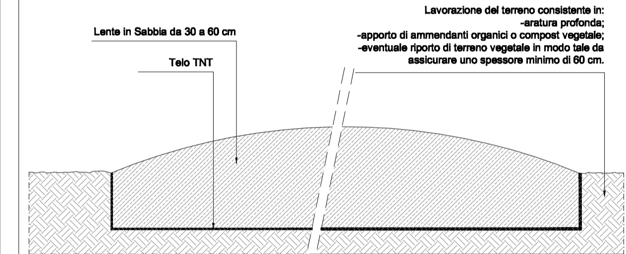
SCALA 1:20
