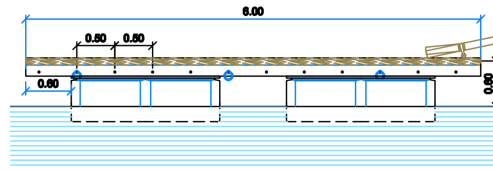
VISTA LATERALE (scala 1:50)
