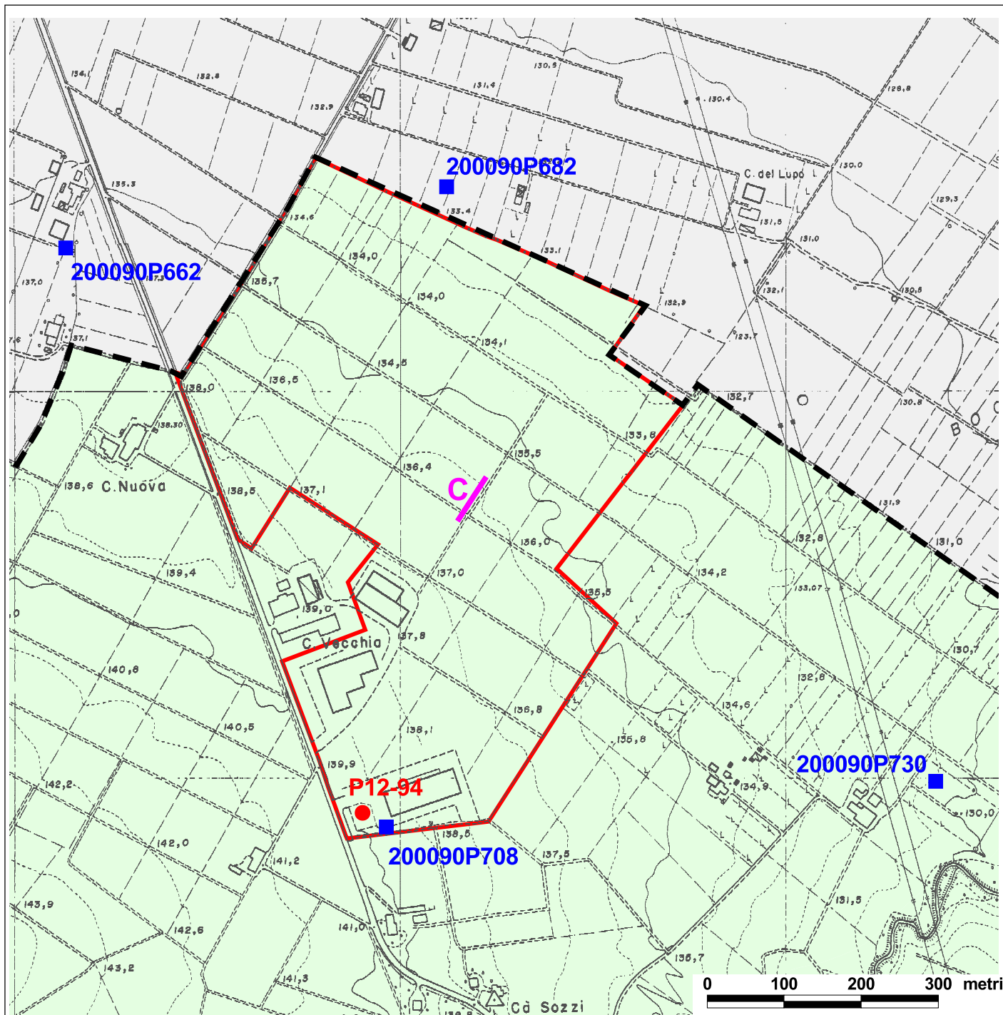
TAV. 4c - CARTA DELLE INDAGINI GEOGNOSTICHE
